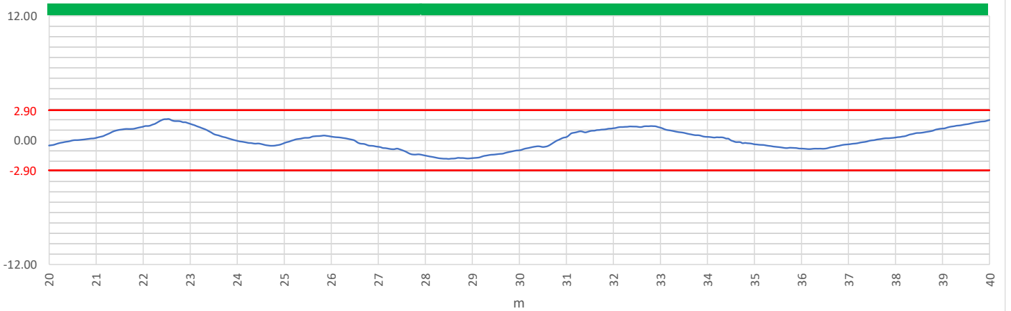
A1 - Longitudinal Levelness (dL)
